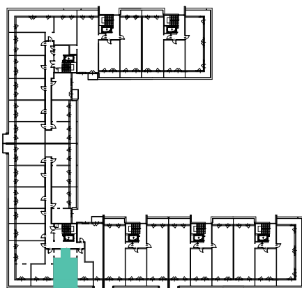
RZUT KONDYGNACJI
